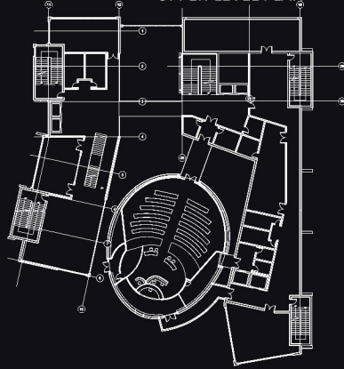
UPPER-LEVEL PLAN
